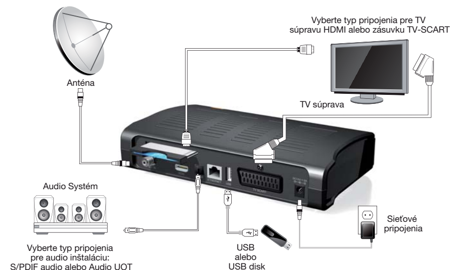
Obr. č. 3 – schéma zapojenia Set-top boxu.
