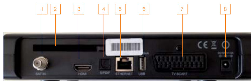
Obr. č. 2 - zadná strana Set-top boxu.
